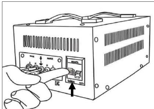
Рис. 13. Включение байпаса
