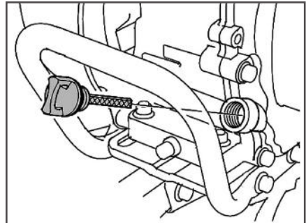
Рис. 18 Крышка-щуп маслозаливной горловины
