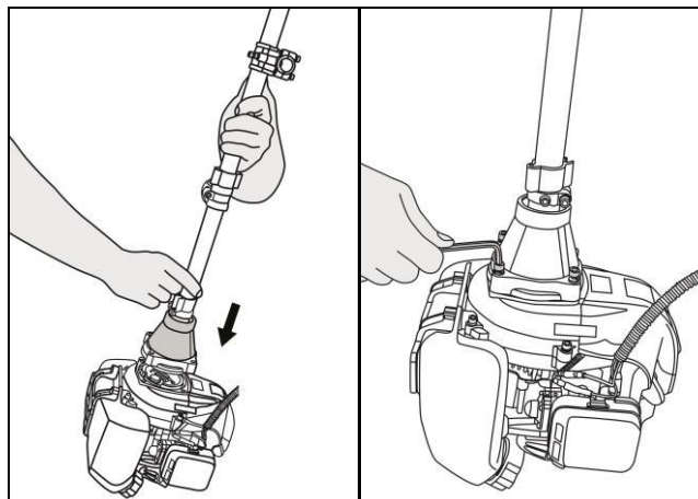
Рис. 6. Установка штанги
