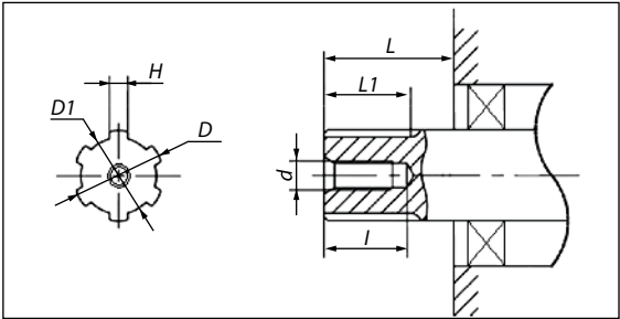
Рис. 4. Выходной вал двигателя RX-17K
