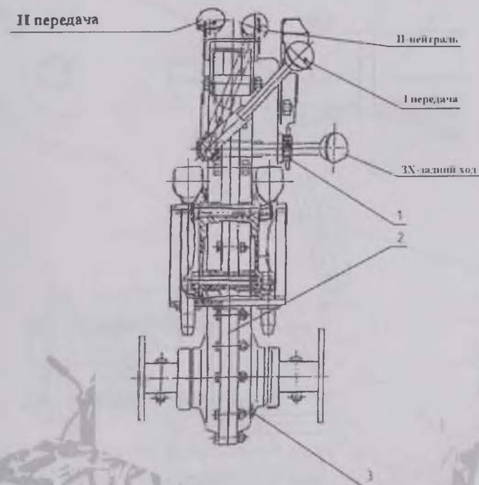
Рис. 5 Редуктор мотоблока
