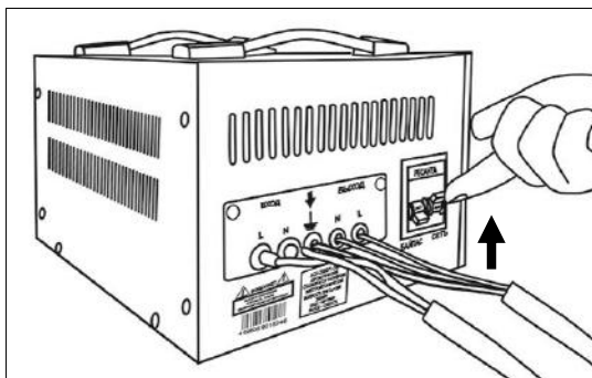
Рис 11. Включение стабилизатора
