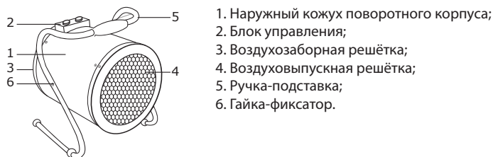
Рис. 1. Устройство прибора
