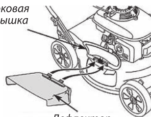
Дефлектор
