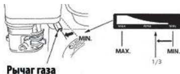
Рычаг газа
