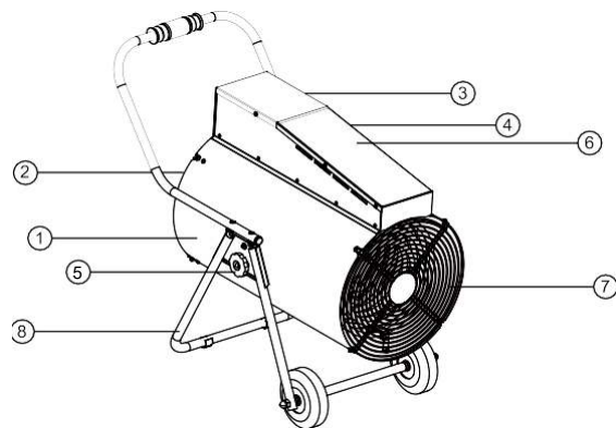
Рис. 1.1 Устройство прибора.
