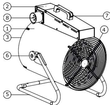
Рис. 1.2 Устройство прибора.
