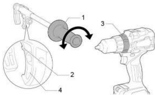
1. Рукоятка 2. Паз
