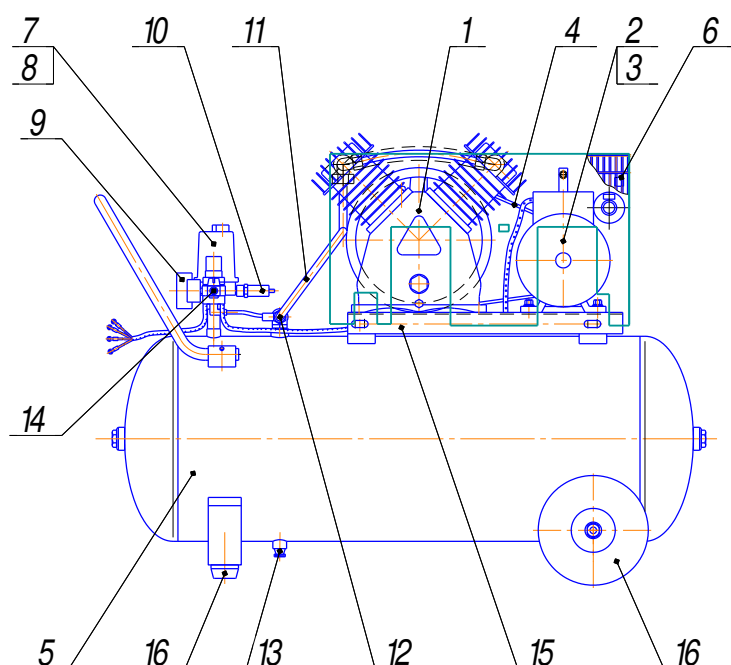
Рисунок 7 - Общий вид компрессоров СБ4/С-100.LB30, СБ4/С-100.LB30А
