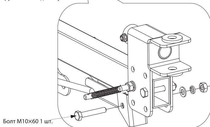
Рис. 12. Схема сборки балки прицепной. Крепление подножки к балке прицепной.
