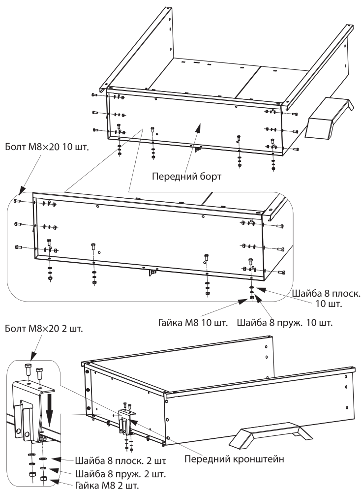
Рис. 3. Схема сборки кузова. Сборка борта переднего и переднего кронштейна.
