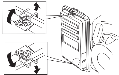
Рис. 8. Снятие крышки воздушного фильтра
