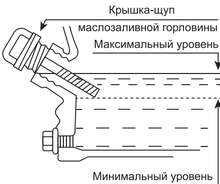
Рис. 6 Проверка уровня масла в картере
