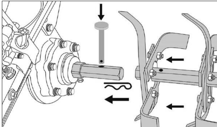
Рис. 6. Установка фрезы
