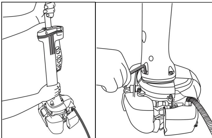
Рис. 6. Установка штанги
