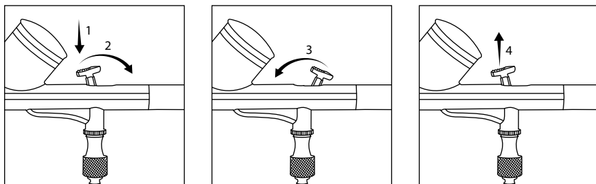
Рис. 4. Аэрограф двойного независимого действия
