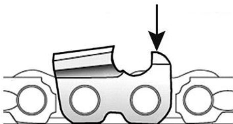
Рис. 19 Ограничитель глубины резания
