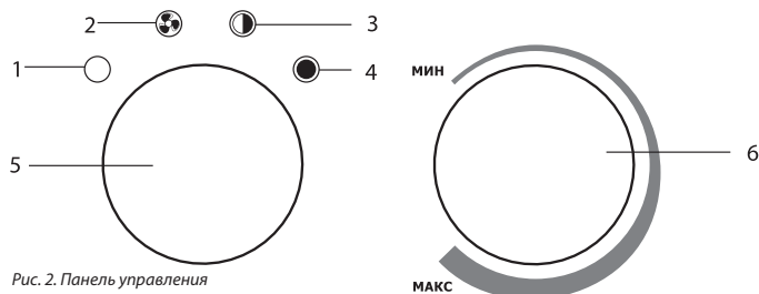
Рис. 2. Панель управления
