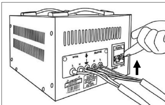
Рис 11. Включение стабилизатора
