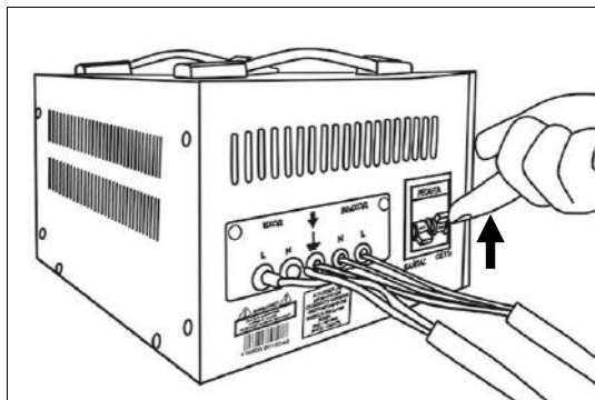
Рис. 8. Включение стабилизатора
