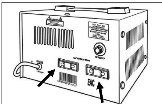
Рис. 5. Подключение нагрузки
