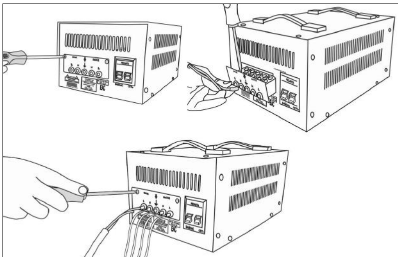
Рис 10. Подключение стабилизатора через клеммную колодку
