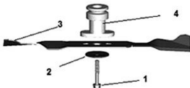
Рис. 18 Обслуживание ножа
