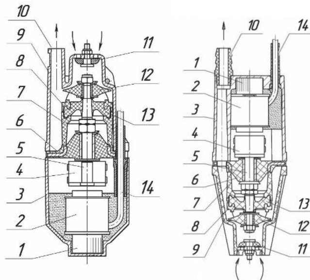
Рис. 1 Верхний забор воды
