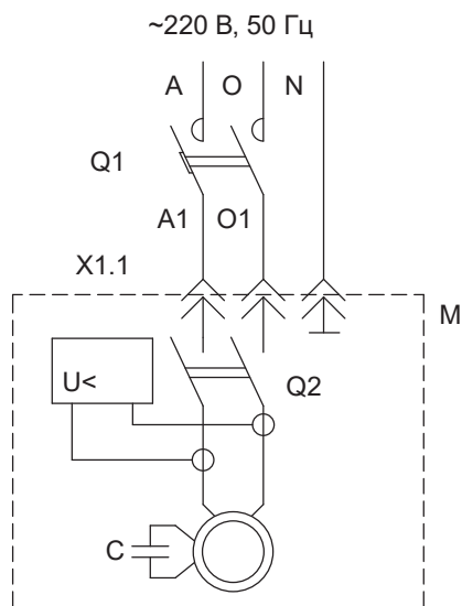
Схема электрическая принципиальная для В-160, В-180
