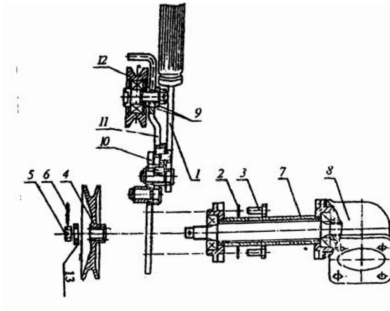
Рис. 4. Натяжное устройство
