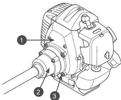
Рис. 5 Установка двигателя
