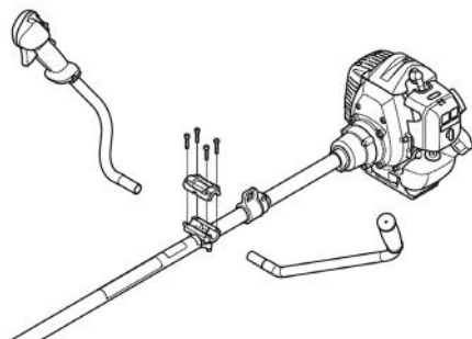
Рис. 6 Установка рукояток
