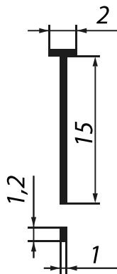
Т-образный гвоздь
