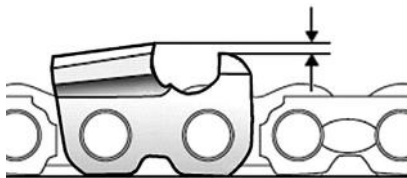
Рис. 22 Глубина резания
