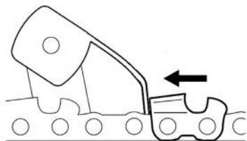
Рис. 20 Упор цепи
