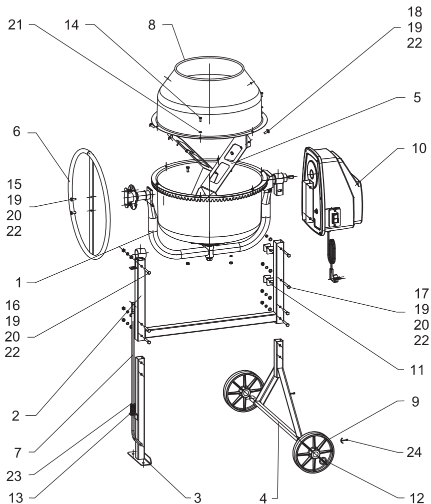
Рис. 1 BCE-120 (вид с разнесенными элементами)
