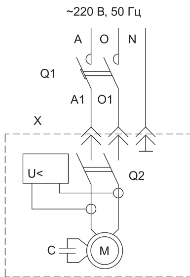
Схема электрическая принципиальная для БСЕ-160, БСЕ-180
