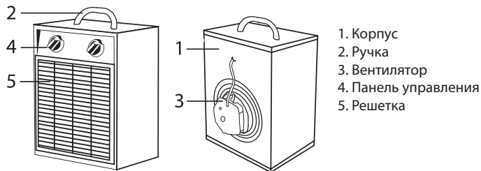
Рис. 1. Устройство прибора
