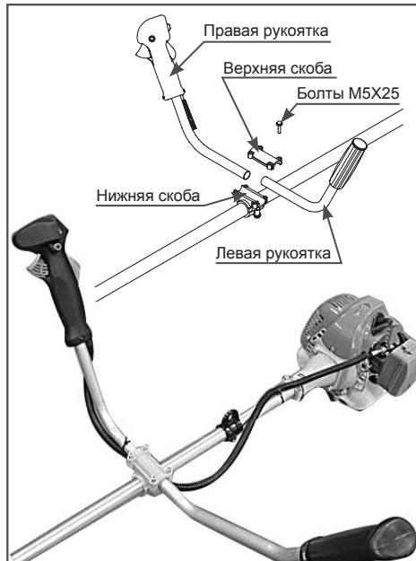
Рис. 4 Установка рабочей рукоятки
