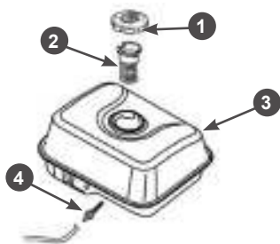
Рис. 39 Фильтры топливные
