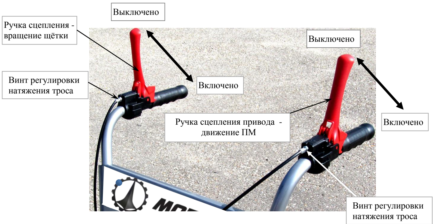
РИС. 4 СХЕМА ВКЛЮЧЕНИЯ РУЧЕК СЦЕПЛЕНИЯ
