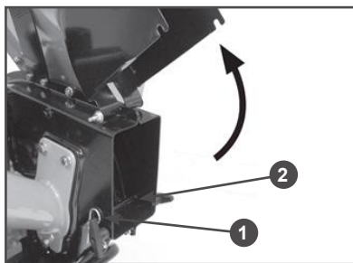
Рис. 18 Разблокировка решетки разгрузочной трубы
